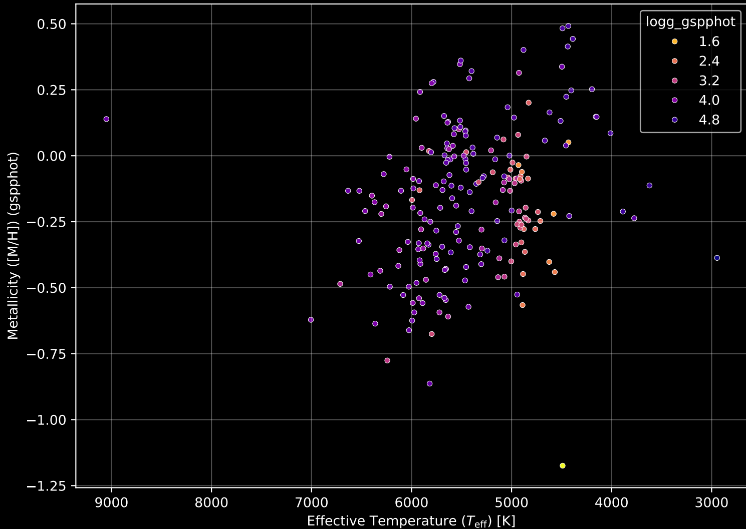
APOGEE DR17 Field: [269-37-O_TESS] Stellar Population Parameters (n= 212)
